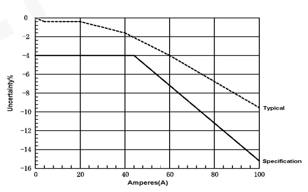
图 4 典型的 DC 线性度 (0.01V/A 档位)
